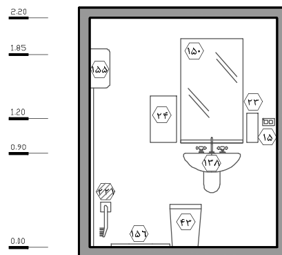
نقشه ۲-۸۰- نما ۴ - مقیاس ۱:۵۰
