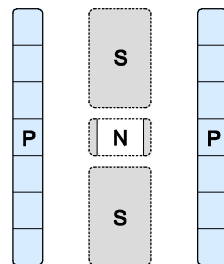
شکل ۲-۱۱- چیدمان H
