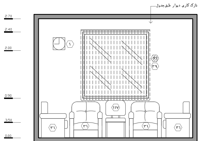
نقشه ۲-۴۸ - نما ۴ - مقیاس ۱:۵۰
