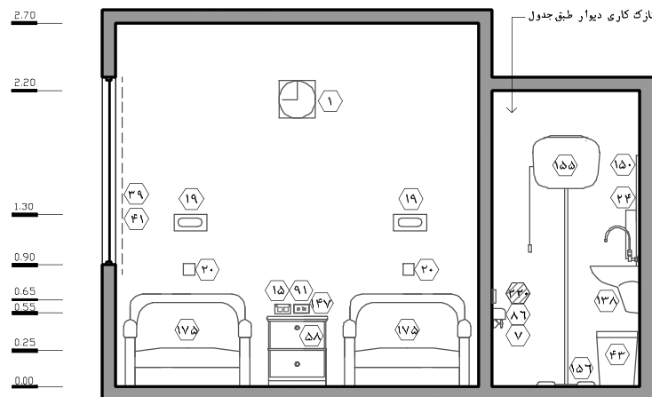
نقشه ۲-۷۹- نما ۳ - مقیاس ۱:۵۰
