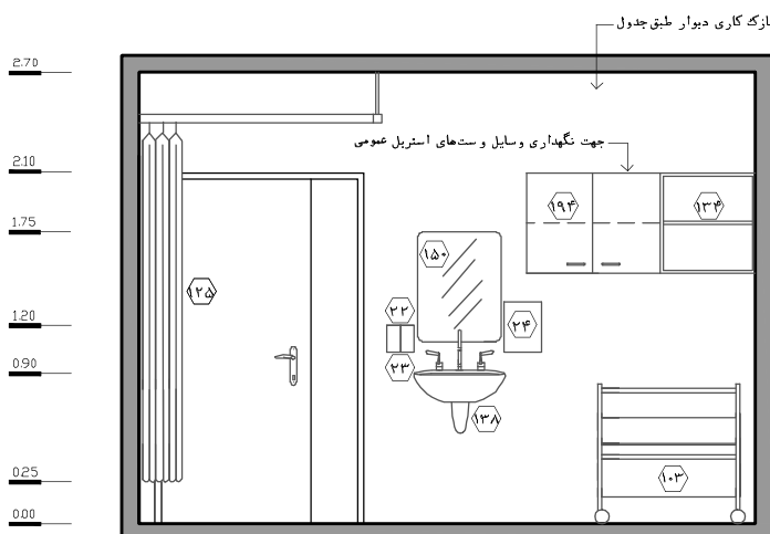
نقشه ۲-۲۸ - نما ۲ - مقیاس ۱:۵۰
