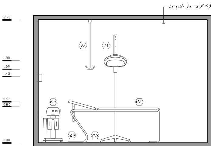
نقشه ۲-۲۹ - نما ۳ - مقیاس ۱:۵۰
