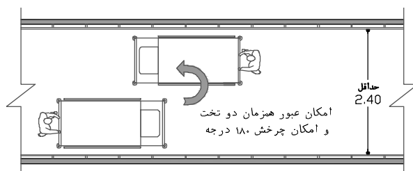
نقشه ۲-۹۸- راهرو با عرض حداقل ۲/۴ متر جهت عبور همزمان دو تخت بستری از کنار یکدیگر و امکان چرخش ۱۸۰ درجه مقیاس ۱:۱۰۰
