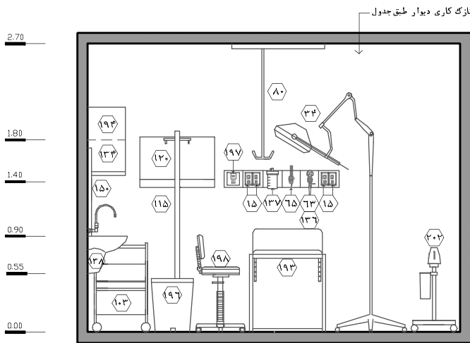
نقشه ۲-۲۷ - نما ۱ - مقیاس ۱:۵۰
