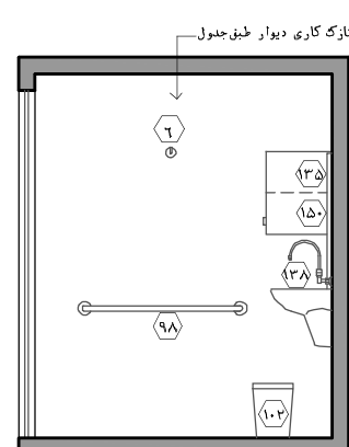
نقشه ۲-۹۱- نمای ۲ - مقیاس ۱:۵۰
