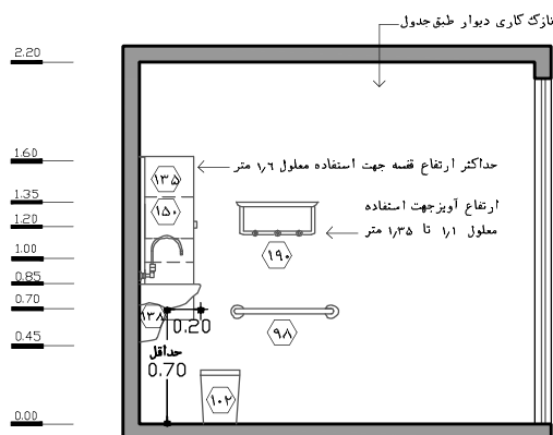
نقشه ۱-۹۳- نمای ۱- مقیاس ۱:۵۰
