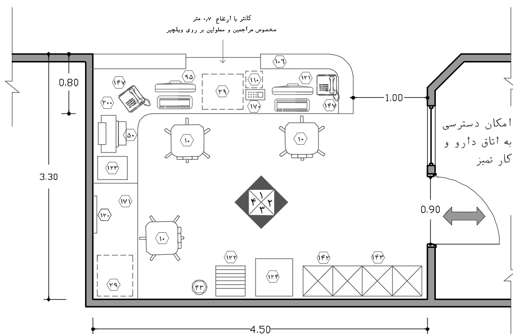
نقشه ۲-۳۰ - پلان ایستگاه پرستاری - مقیاس ۱:۵۰
