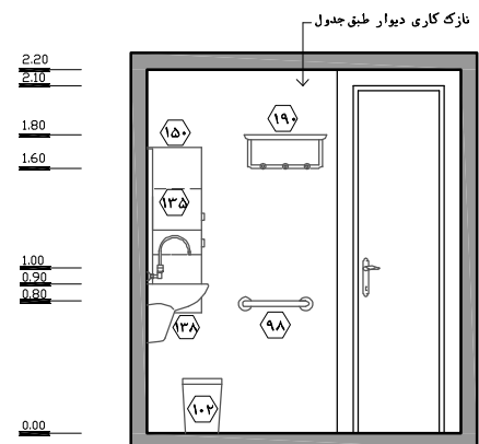
نقشه ۲-۱۲- نما ۱- مقیاس ۱:۵۰
