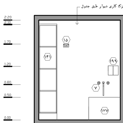
نقشه ۲-۷۱- نما ۳ - مقیاس ۱:۵۰
