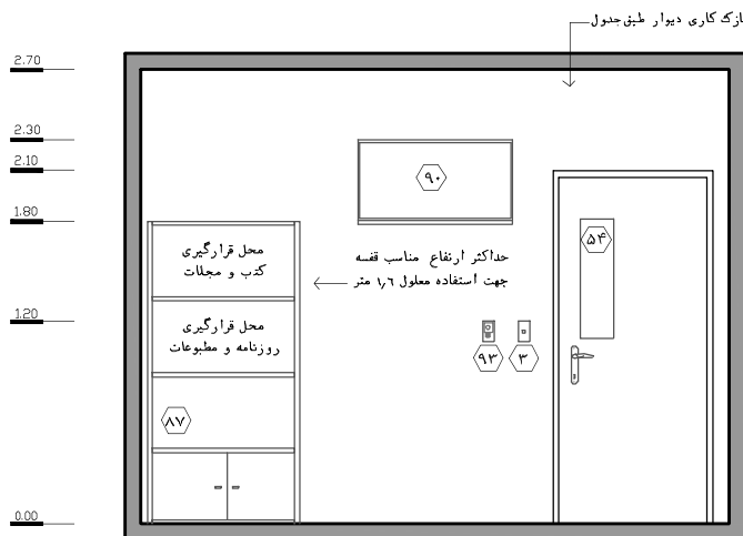
نقشه ۲-۴۷ - نما ۳ - مقیاس ۱:۵۰
