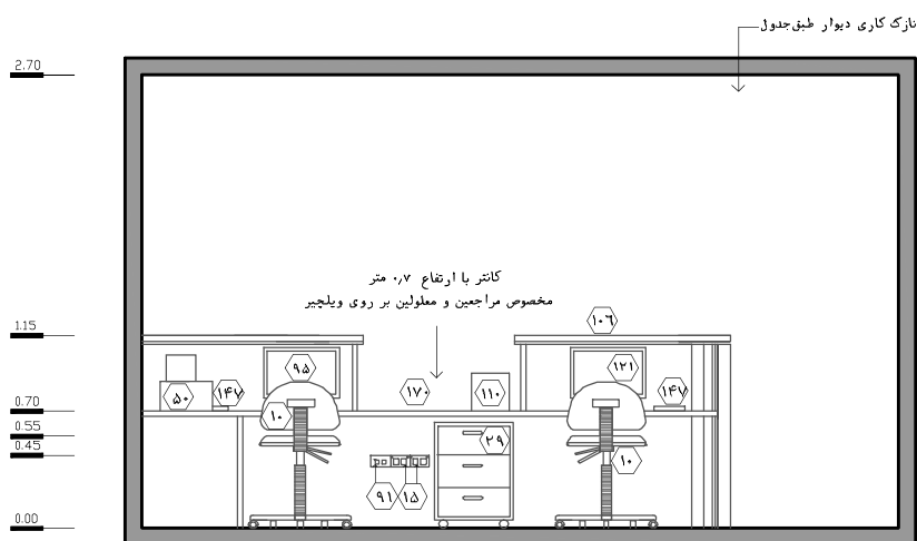
نقشه ۲-۳۱ - نما ۱ - مقیاس ۱:۵۰
