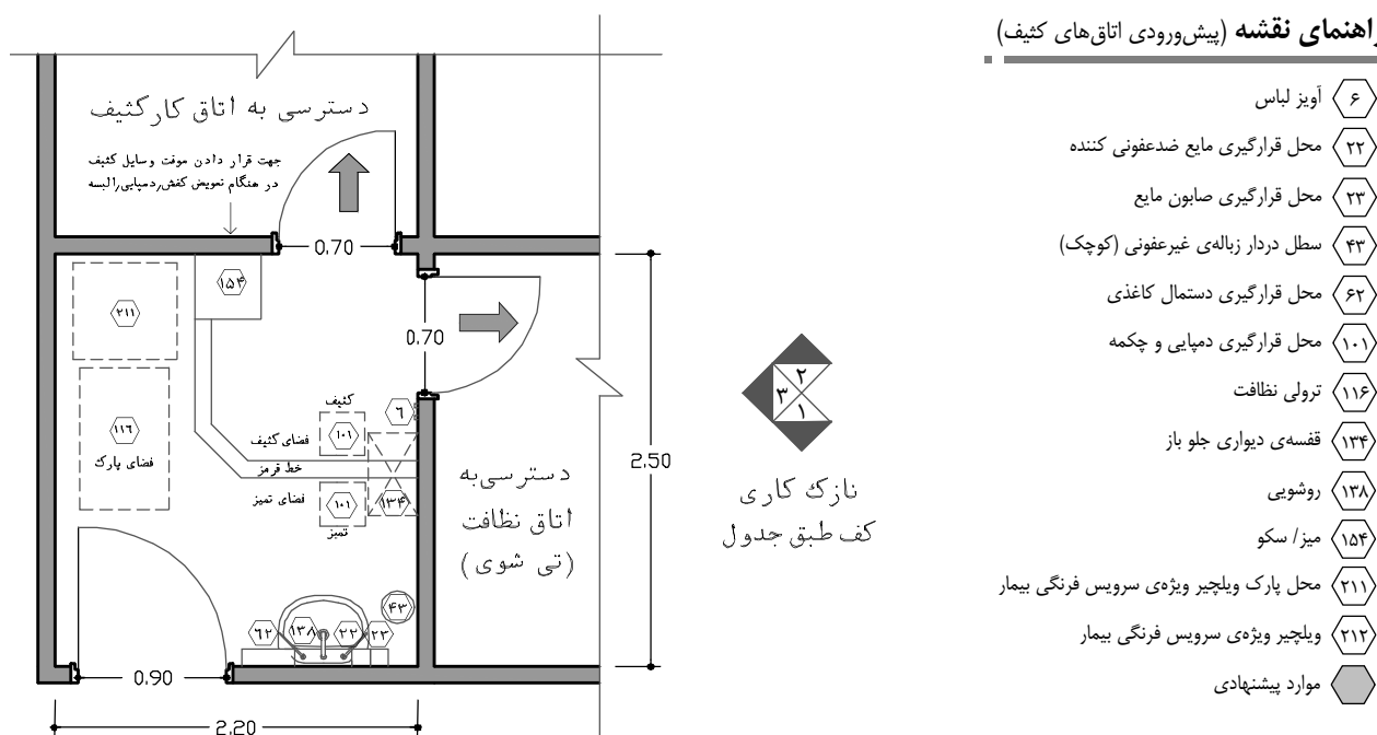
نقشه ۲-۵۷- پلان پیش‌ورودی اتاق کار کثیف - مقیاس ۱:۵۰
