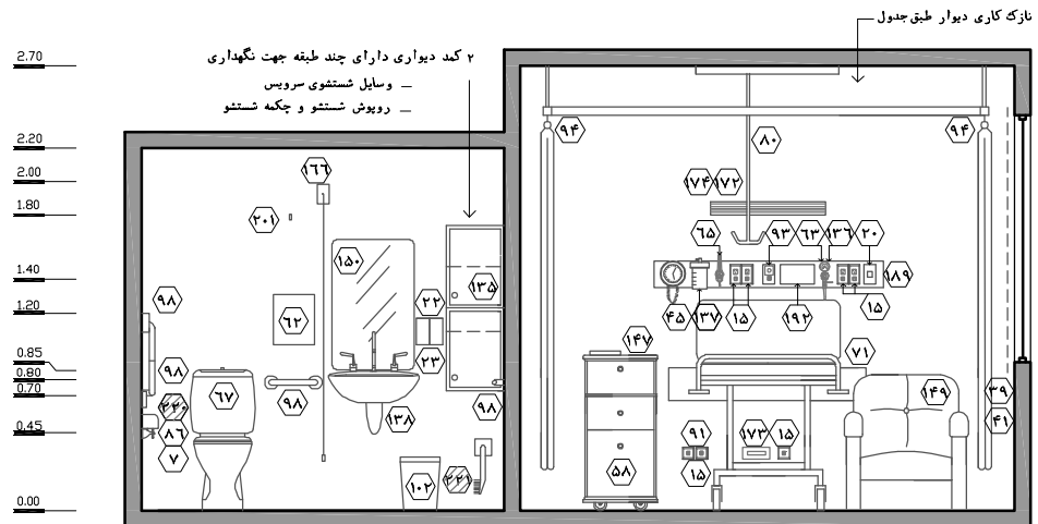
نقشه ۲-۴ - نما ۳ - مقیاس ۱:۵۰
