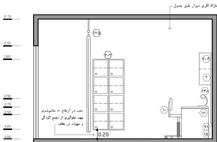
نقشه ۲-۷۸- نما ۲ - مقیاس ۱:۵۰
