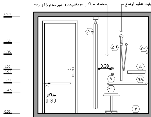
نقشه ۴-۹۶- نمای ۴- مقیاس ۱:۵۰
