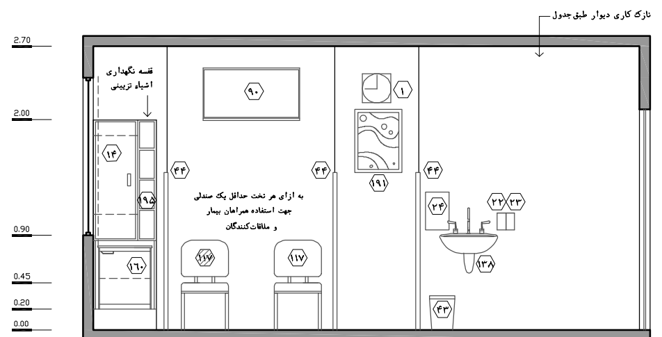
نقشه ۲-۶ - نما ۵ - مقیاس ۱:۵۰
