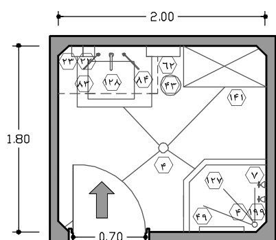
نقشه ۲-۶۸- پلان اتاق نظافت (تی‌شوی) - مقیاس ۱:۵۰
