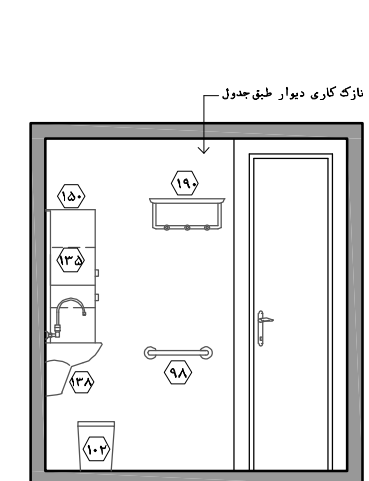
نقشه ۲-۵ - نما ۴ - مقیاس ۱:۵۰
