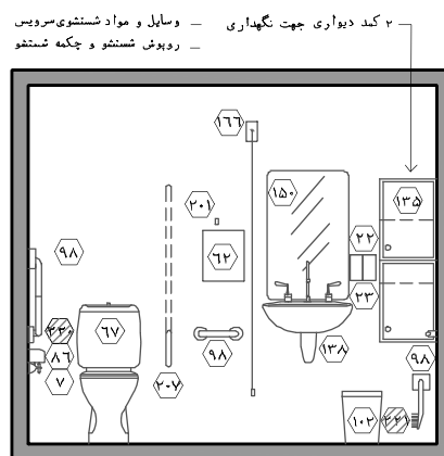
نقشه ۲-۹۴- نمای ۲- مقیاس ۱:۵۰
