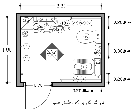
نقشه ۲-۸۸- پلان سرویس بهداشتی عمومی - مقیاس ۱:۵۰
