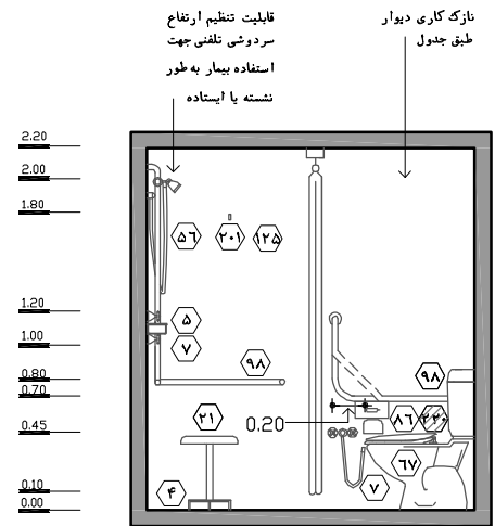
نقشه ۲-۱۳ - نما ۳- مقیاس ۱:۵۰
