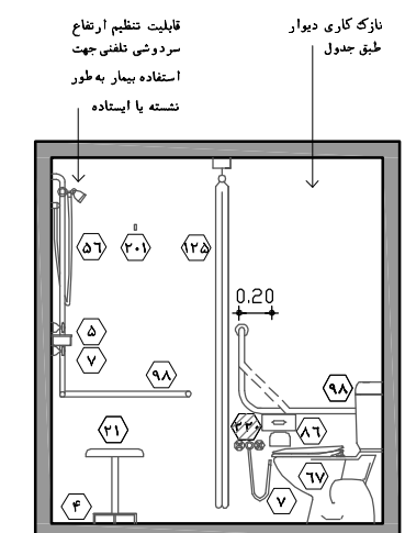
نقشه ۲-۷ - نما ۶ - مقیاس ۱:۵۰
