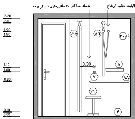
نقشه ۲-۱۰- پلان اتاق بستری دو تخت خوابی مقیاس ۱:۵۰
