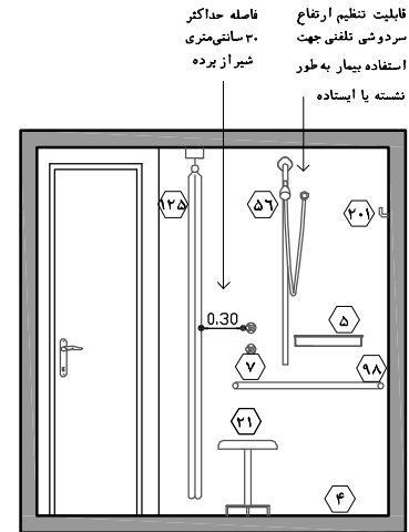
نقشه ۲-۳ - نما ۲ - مقیاس ۱:۵۰
