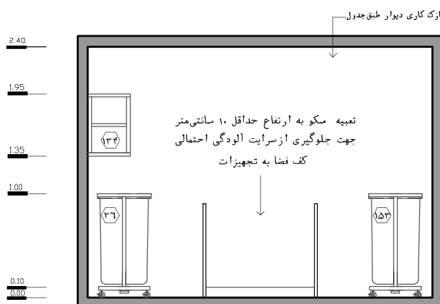
نقشه ۲-۶۷- نما ۱ - مقیاس ۱:۵۰
