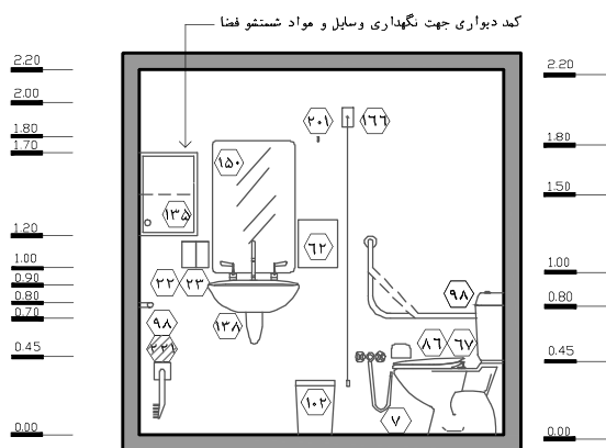
نقشه ۲-۸۹- نمای ۱ - مقیاس ۱:۵۰
