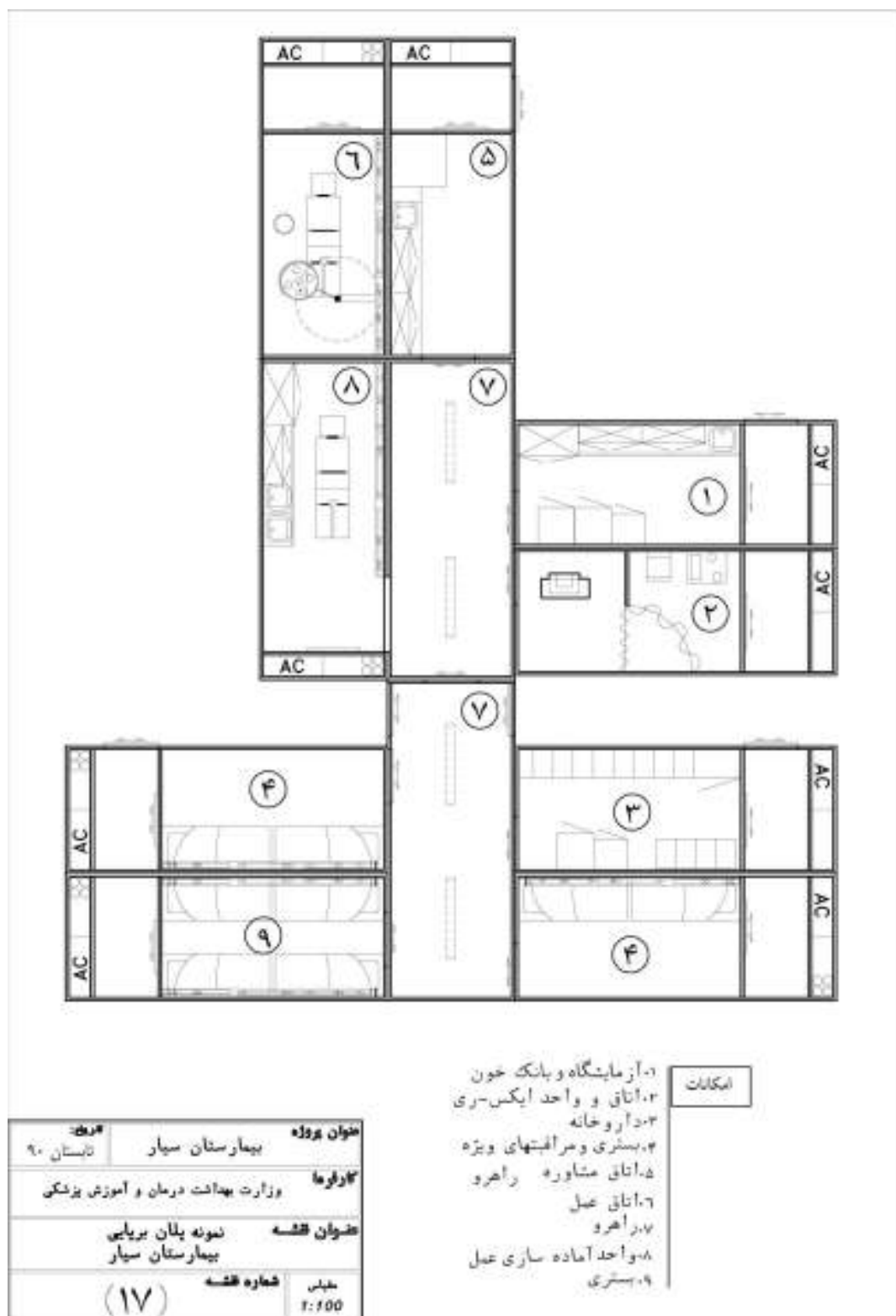
شکل ۱۶-۲ نمونه پلان شماتیک برپایی بیمارستان سیار
