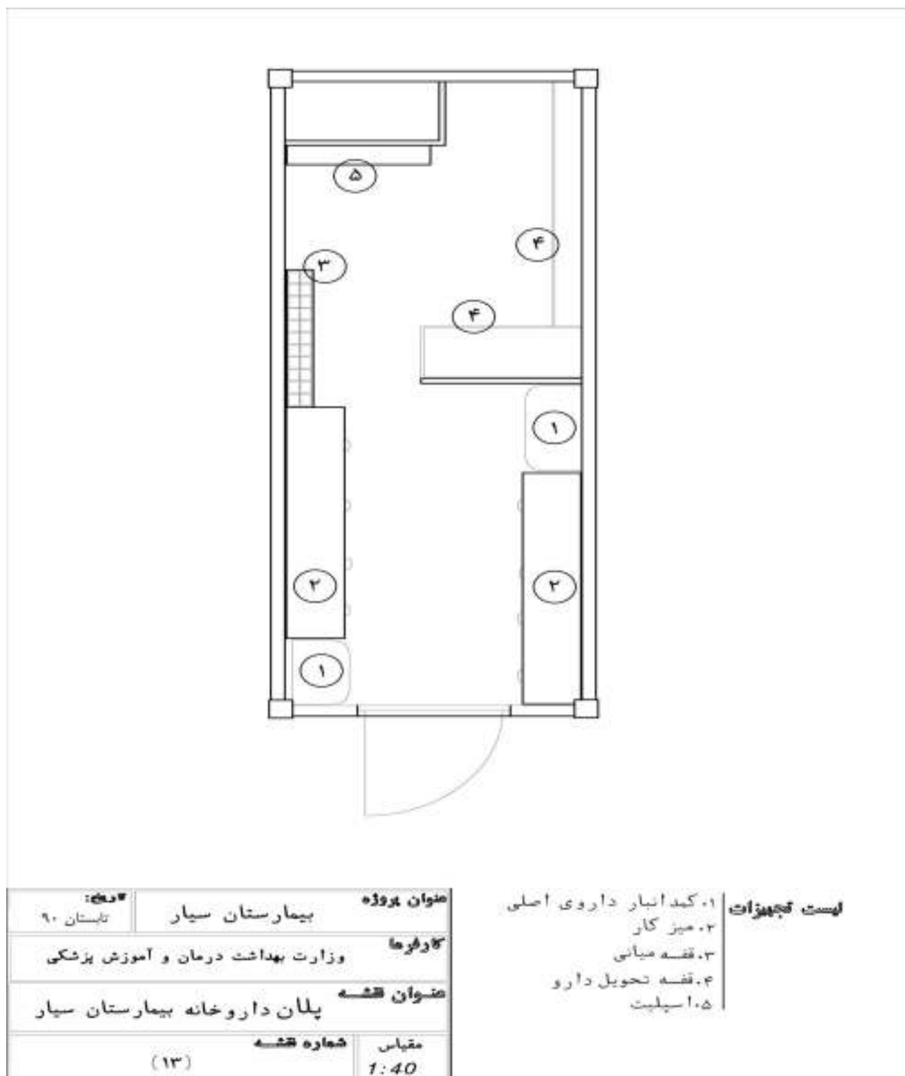
شکل ۸-۲ پلان داروخانه
