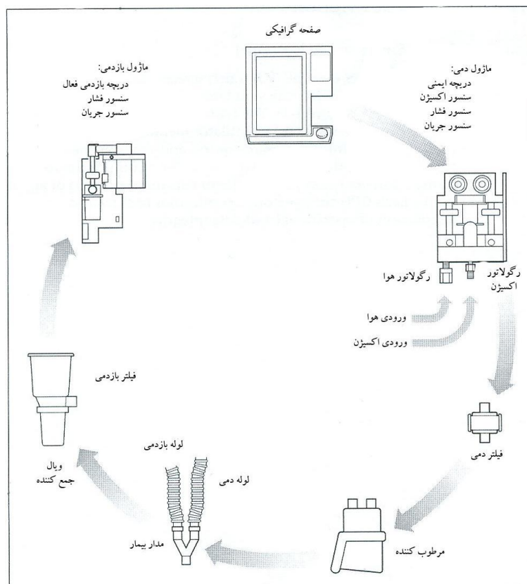
شکل (۱۶) اجزای اصلی یک نوع ونتیلاتور (بنت ۸۴۰) [۳]
