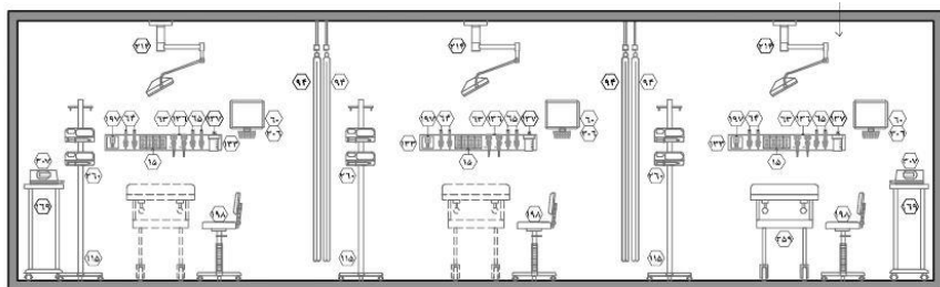
نقشه ی ۲-۱۰۴- نمای ۳- مقیاس ۱:۵۰
