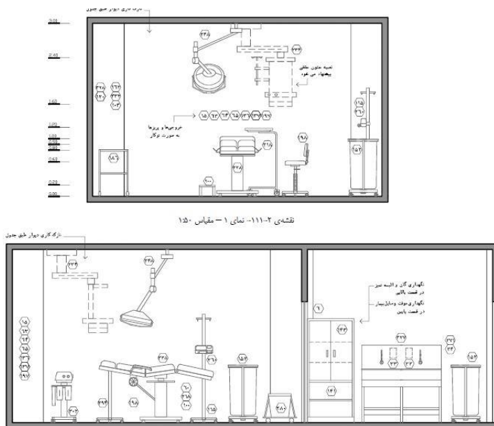
شکل (۳۲): جانمایی اتاق عمل سرپایی بخش اورژانس (وزارت بهداشت، ۱۳۹۰)
