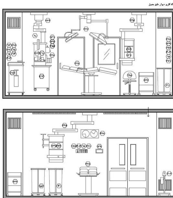
شکل (۴۱): جانمایی فضای اتاق عمل کوچک بخش اعمال جراحی (وزارت بهداشت، ۱۳۹۴)
