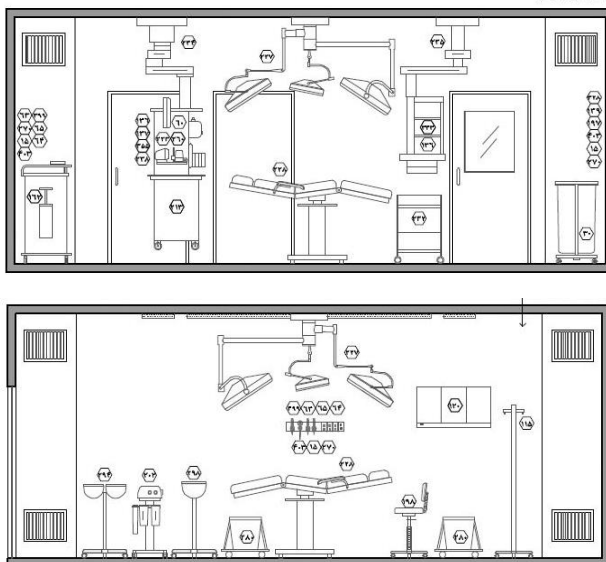
شکل (۴۶): جانمایی فضای اتاق عمل بزرگ بخش اعمال جراحی (وزارت بهداشت، ۱۳۹۴)
