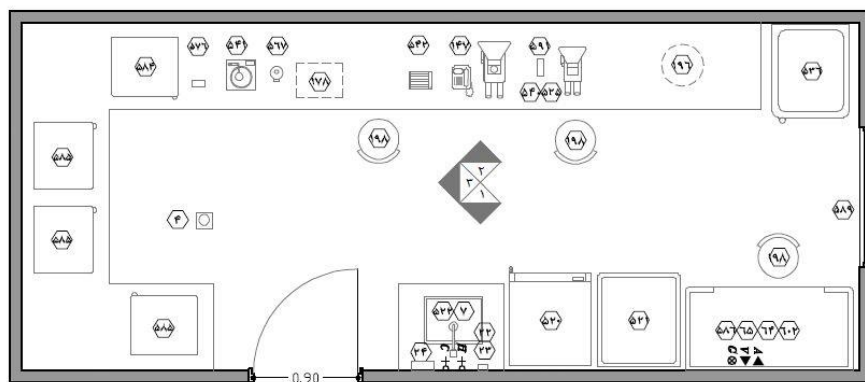
شکل (۶۴): پلان و جانمایی فضای میکروب شناسی بخش آزمایشگاه (وزارت بهداشت، ۱۳۹۴)
