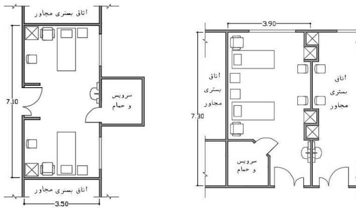
شکل (۱۴): جانمایی تجهیزات پزشکی اتاق دوتخته بخش بستری (وزارت بهداشت، ۱۳۸۹)
