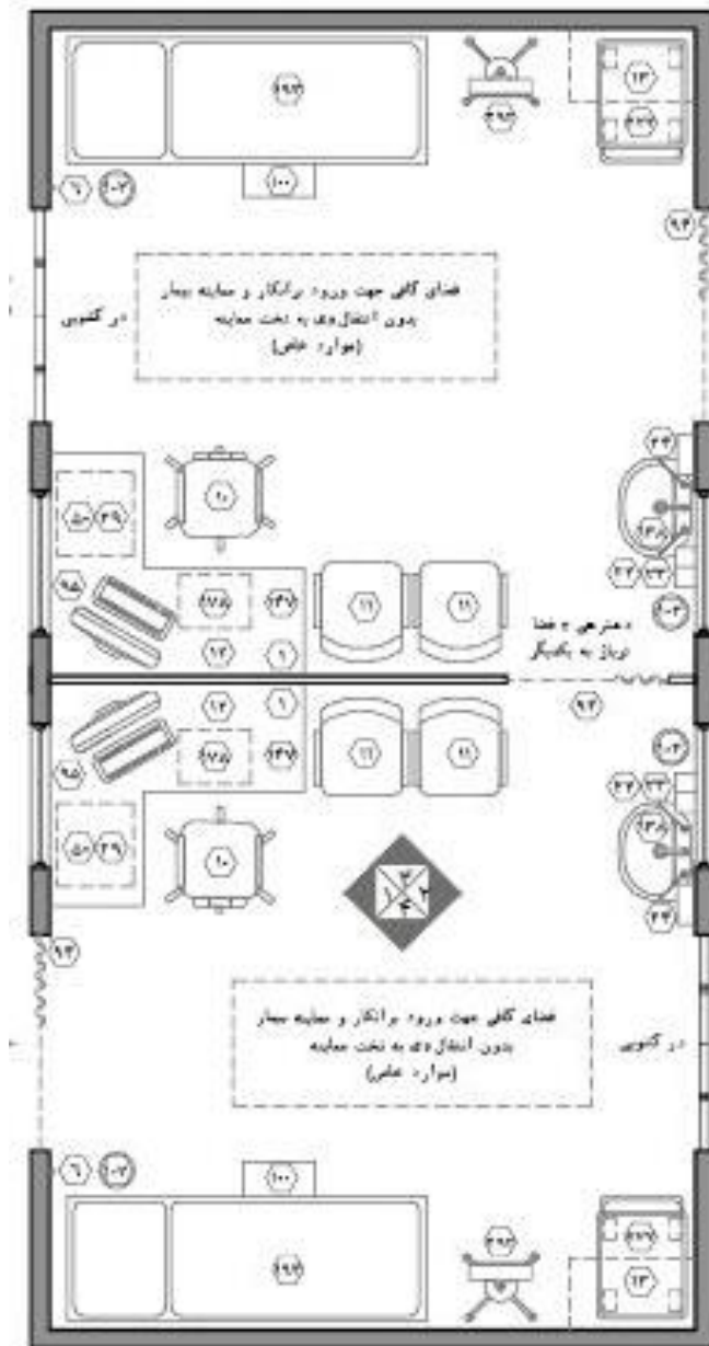
شکل (۲۵): جانمایی فضای تربار بخش اورژانس (وزارت بهداشت، ۱۳۹۰)
