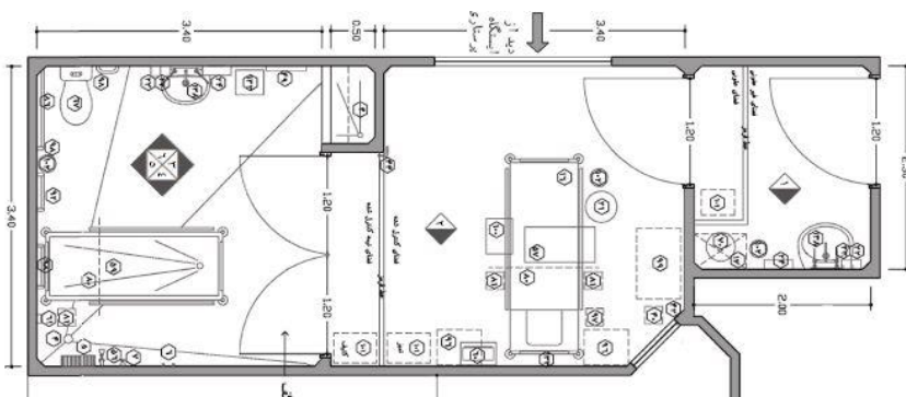
شکل (۲۱): جانمایی تجهیزات پزشکی فضای ایزوله بخش بستری ویژه (وزارت بهداشت، ۱۳۸۸)
